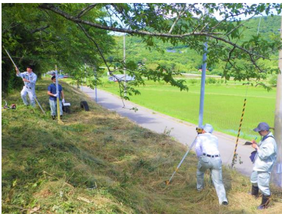
▲ 根岸ため池横断測量の様子
