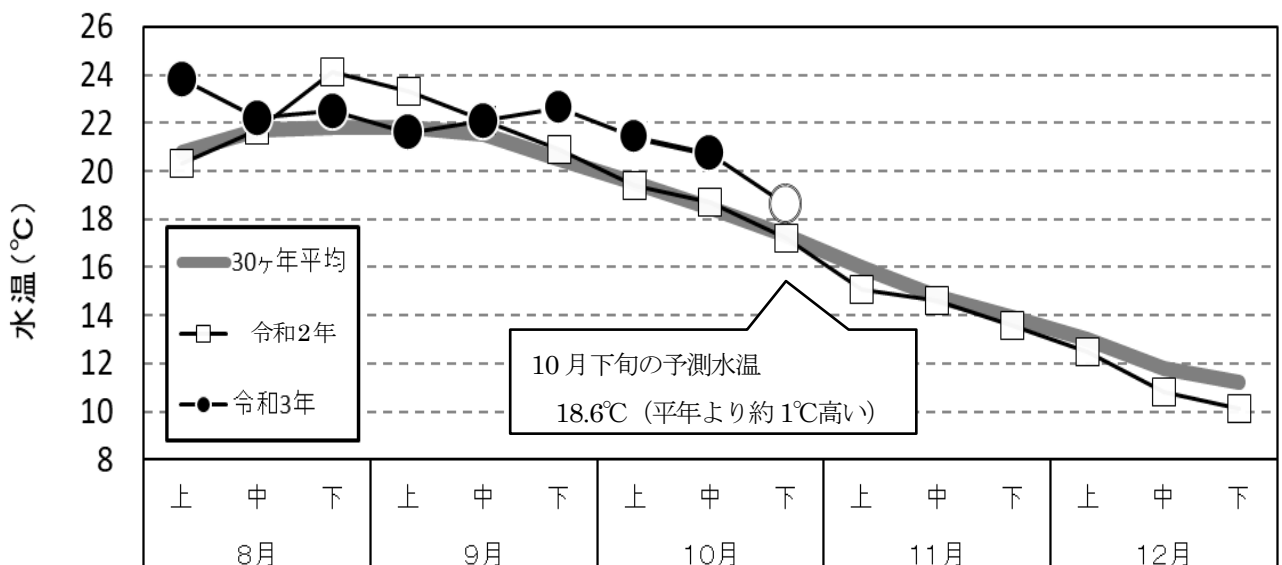
図 気仙沼湾(杉ノ下)表層平均水温の推移
