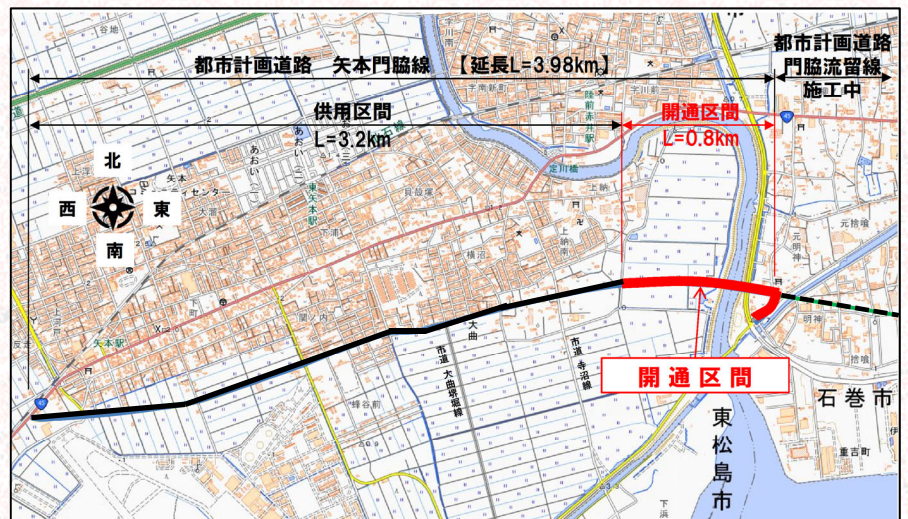
詳細位置図
