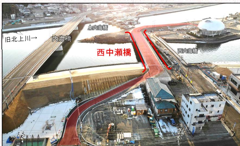
西中瀬橋施工状況(中央地区から望む)
