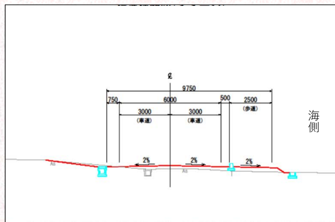
標準断面図 (イメージ)
