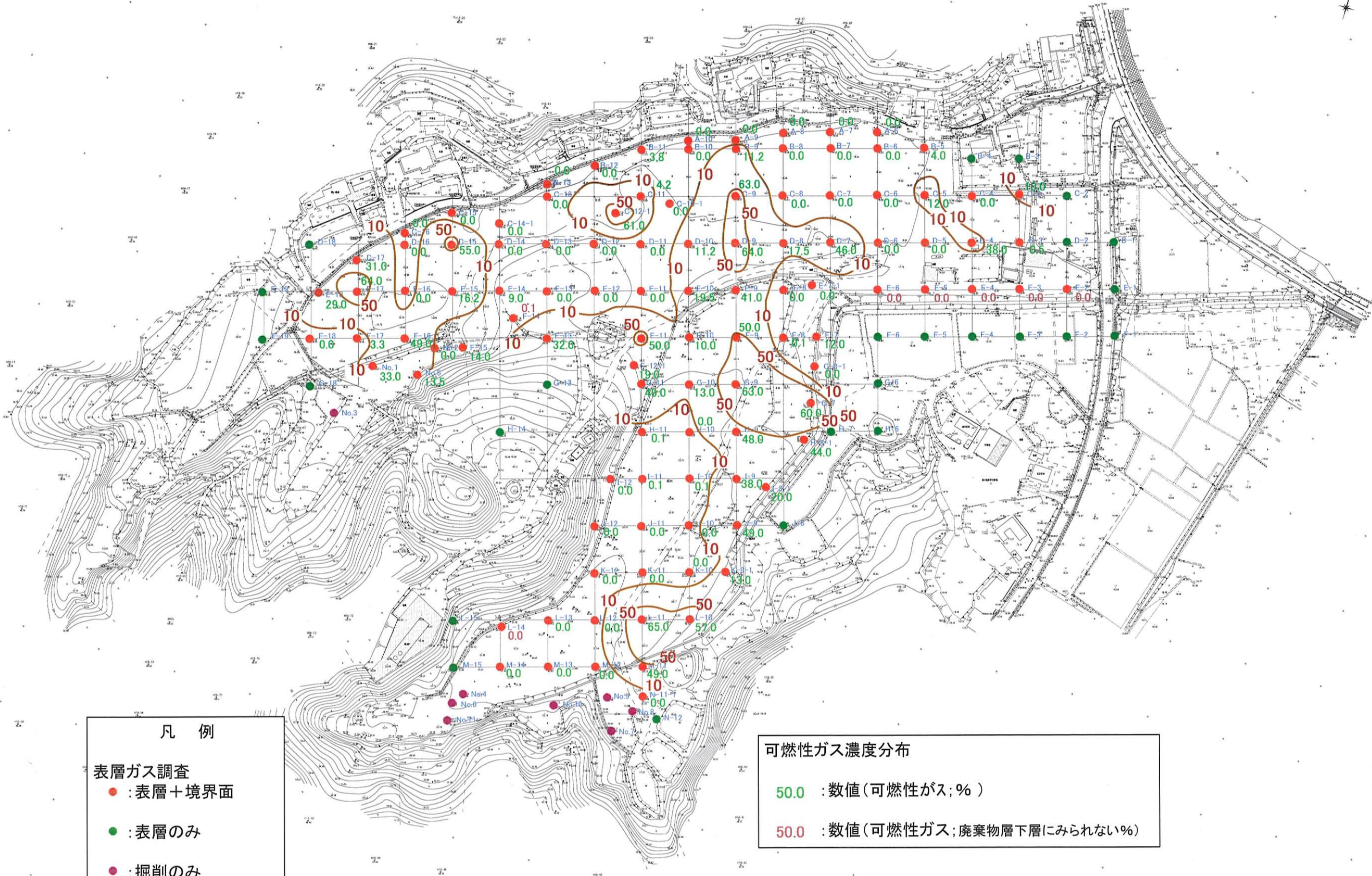
図 1-8 可燃性ガス濃度分布図(覆土/廃棄物層境界面)
