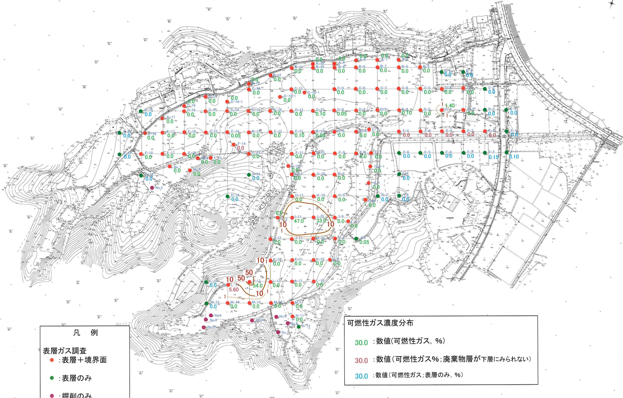
図 1-7 可燃性ガス濃度分布図(表層: 1m深)
