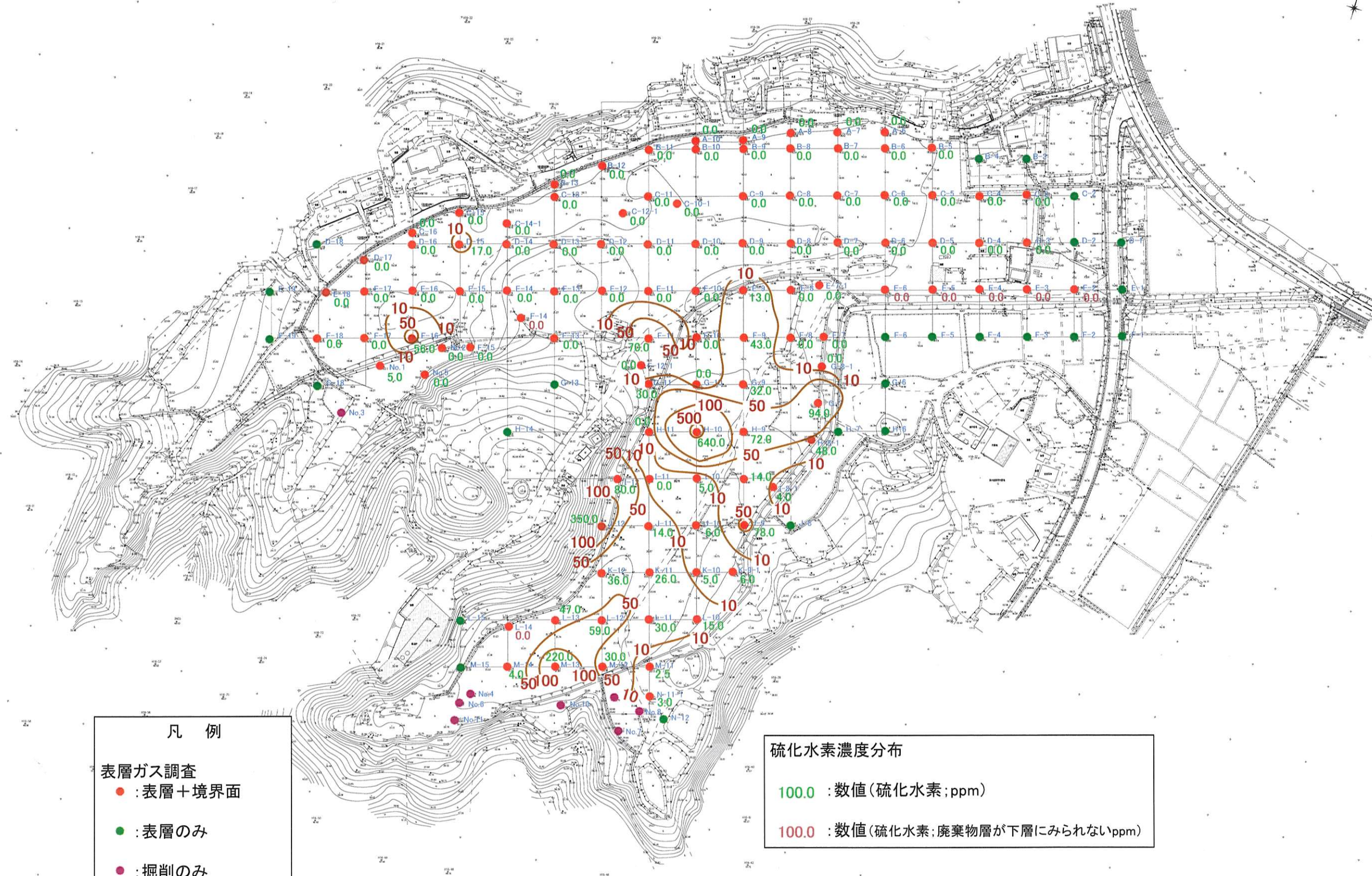
図 1-6 硫化水素濃度分布図(覆土/廃棄物層境界面)
