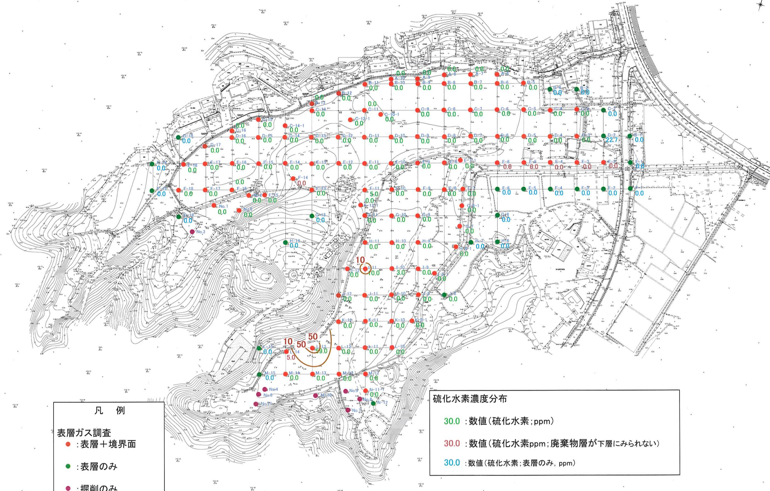
図 1-5 硫化水素濃度分布図(表層: 1m深)
