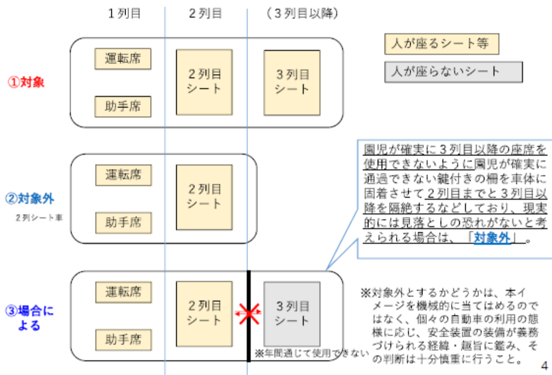
安全装置の装備の義務づけの例外となる自動車のイメージ①
