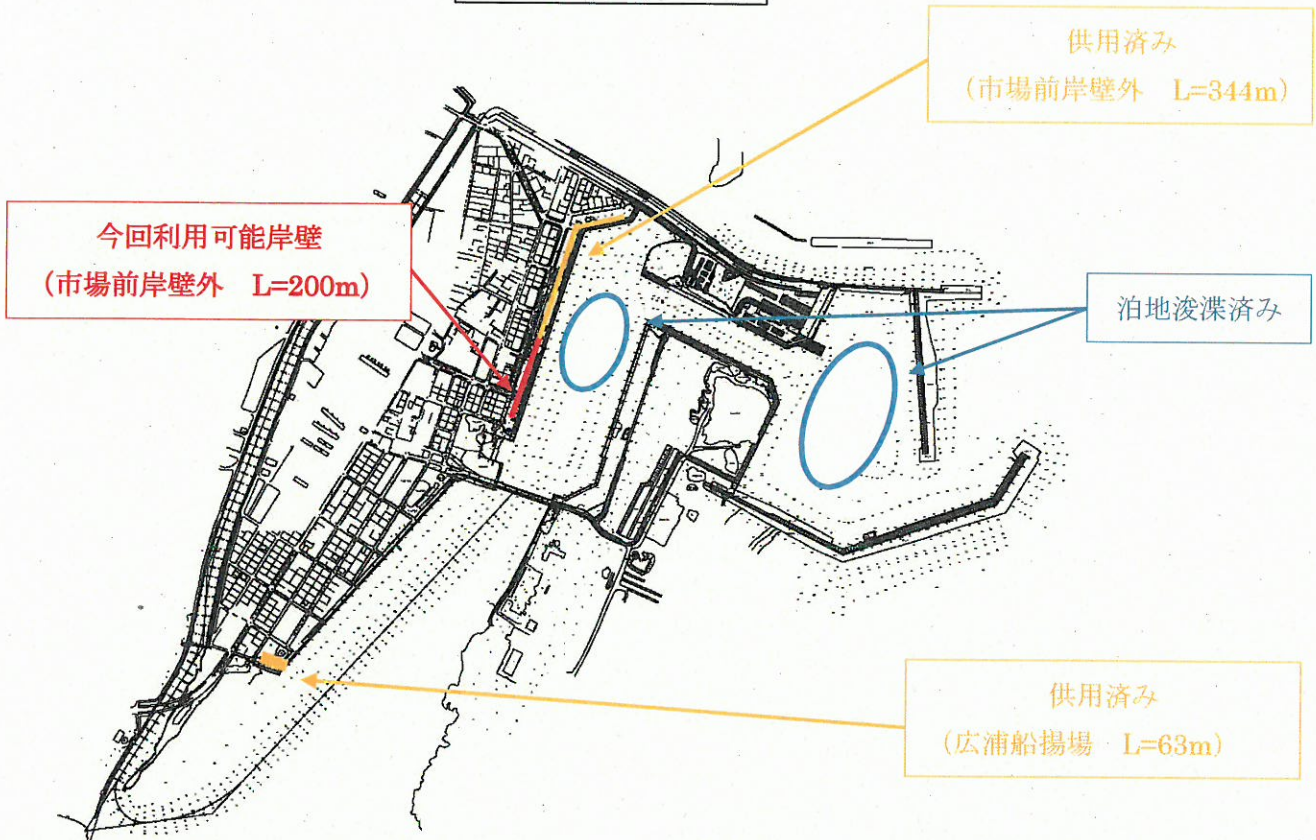
供用済 岸壁 L=344m
