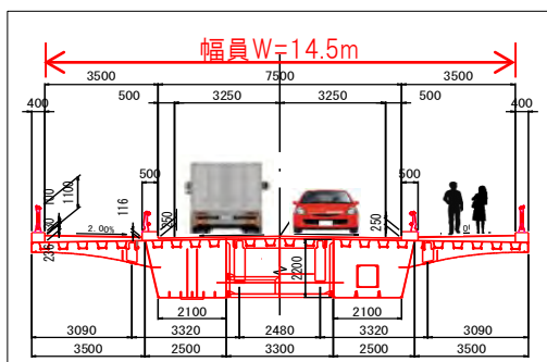
内海橋の断面図
