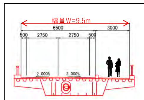
西中瀬橋の断面図
