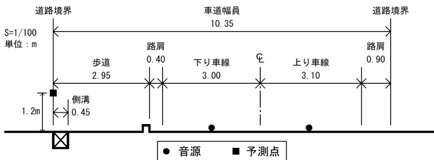
図 6.2.2-8 道路構造, 予測位置及び音源位置
