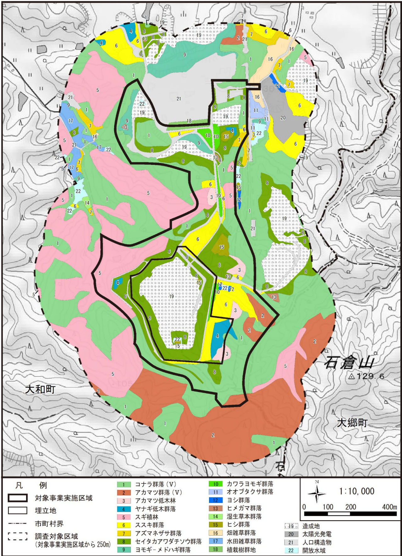
図 6.11.1-3 植生図
