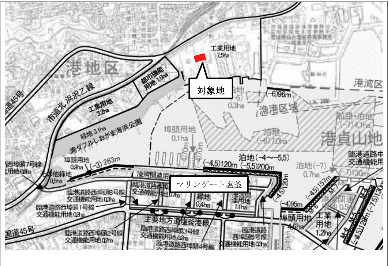
仙台塩釜港（塩釜港区）港湾計画平面図（平成25年改訂）
