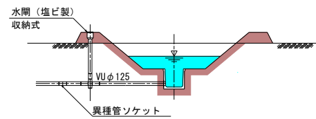
暗渠排水
