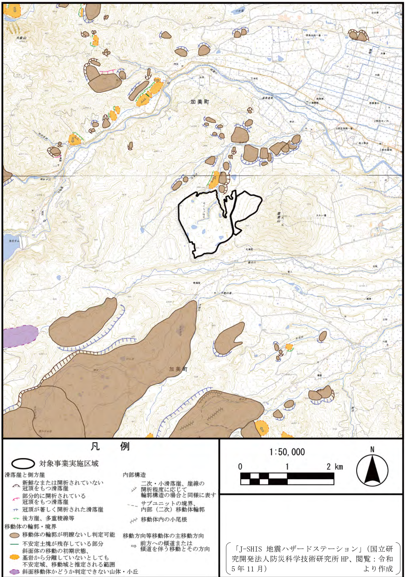
図 3.2-21 地すべり地形の分布
