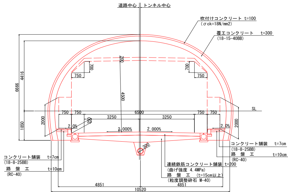
標準断面図 (トンネル部)
