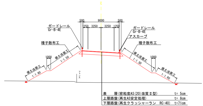
標準断面図 (盛土部)
