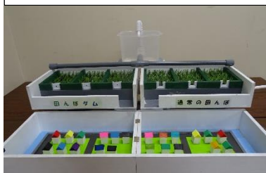
田んぼダム模型製作
