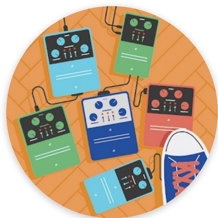
Ras
