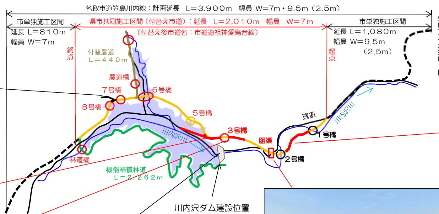
川内沢ダム建設事業全体平面図
