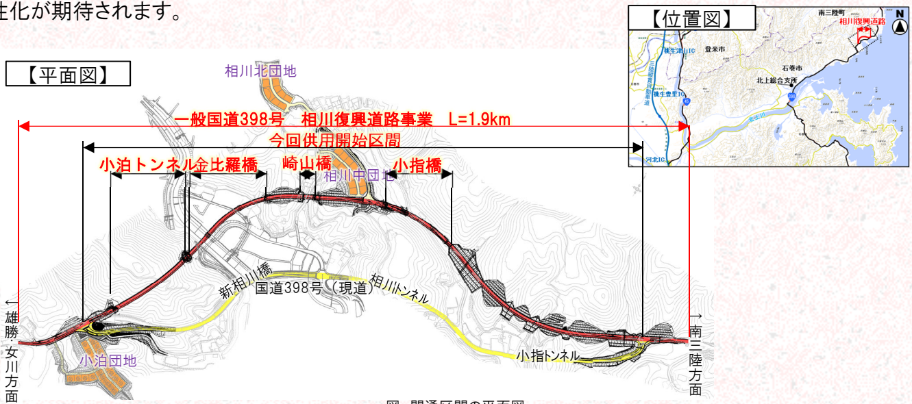
図 開通区間の平面図
