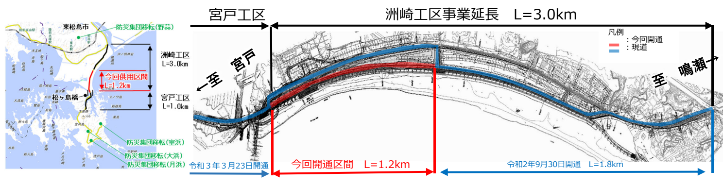
図 開通した洲崎復興道路平面図
