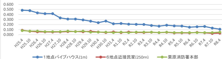
保管庫周辺空間線量推移
