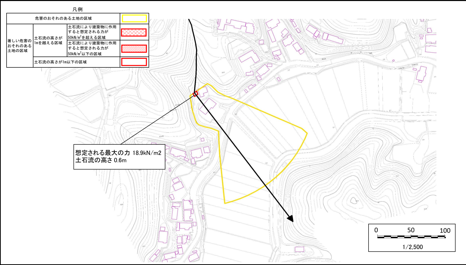
危険のおそれのある土地、著しい危険のおそれのある土地の設定図
