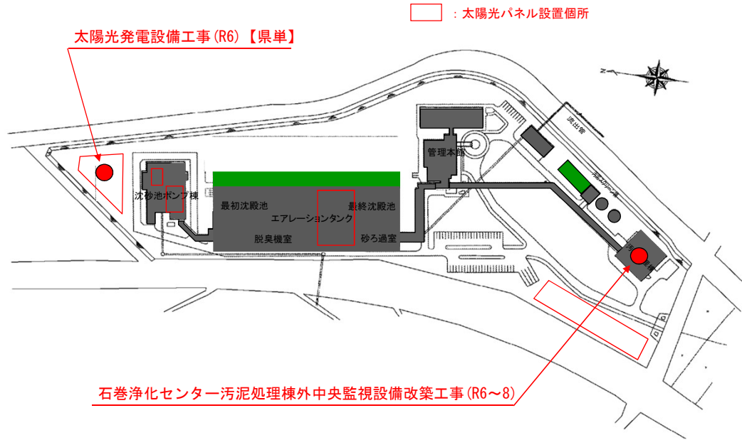
石巻浄化センター一般平面図
