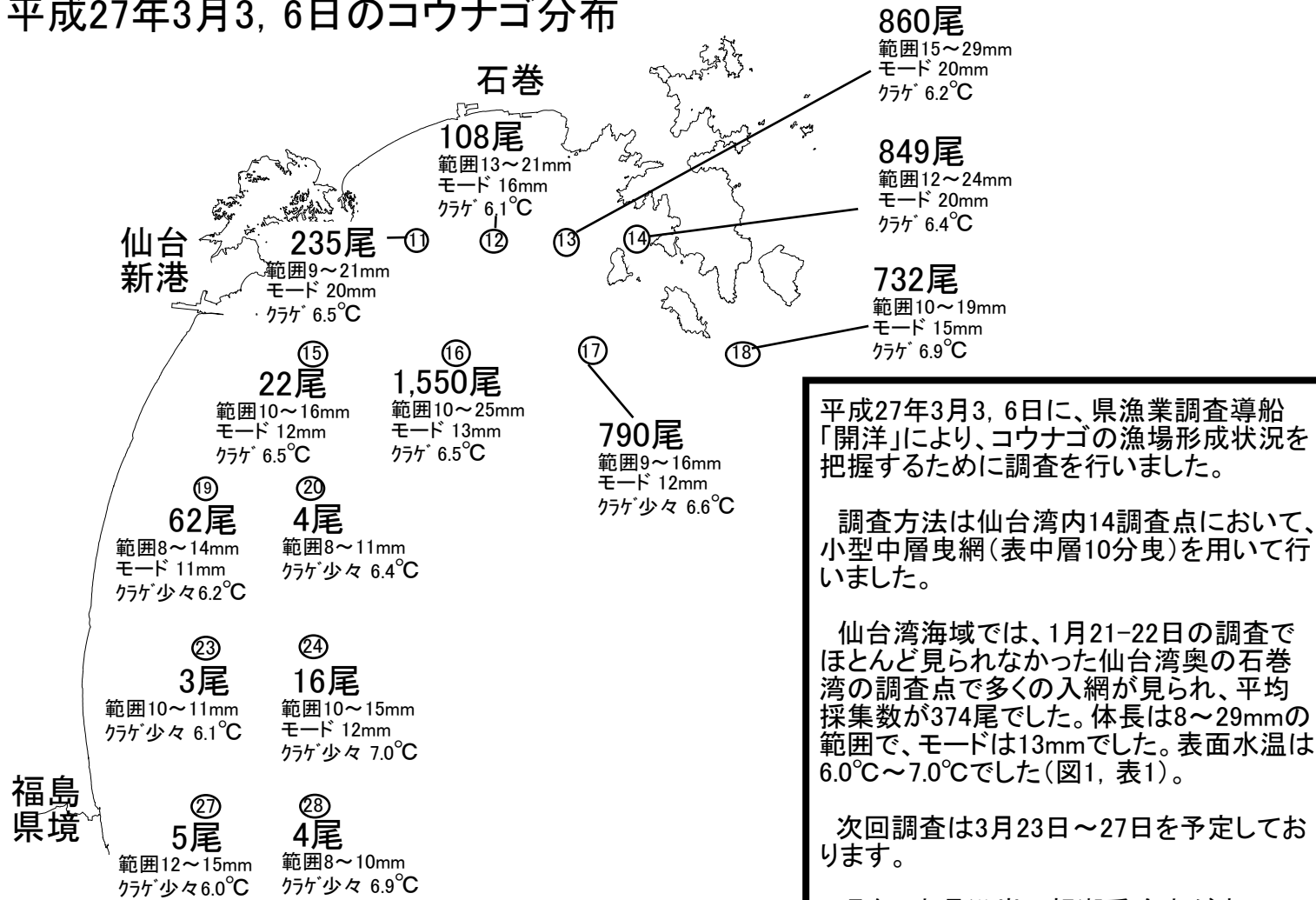
図1 仙台湾分布調査結果(開洋)
