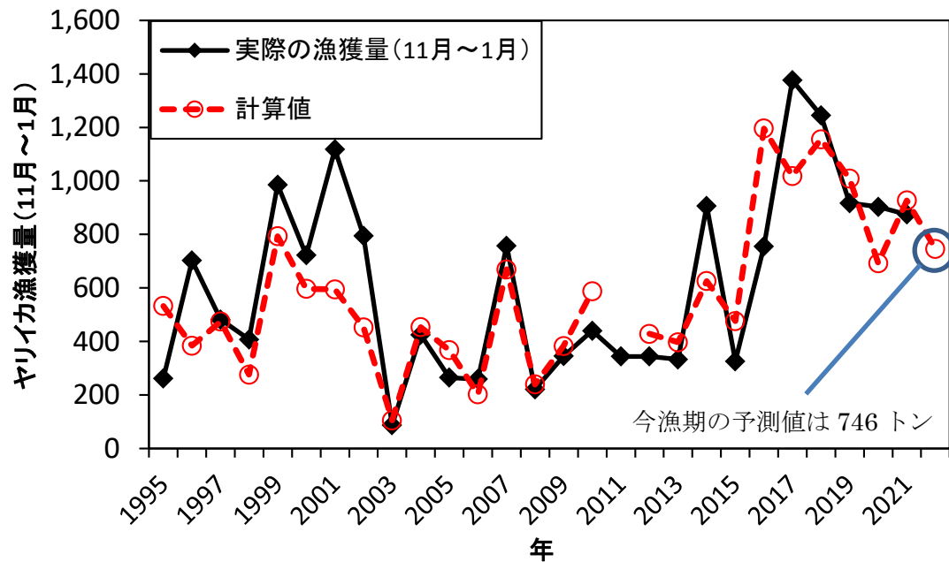
図1 1995年～2022年漁期におけるヤリイカ盛漁期の漁獲量（黒実線）と重回帰分析から得られた計算値（赤色点線）の関係。
