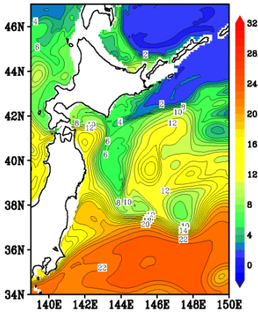
2022 年 11 月上旬/水温/平均値/100m (予報)
