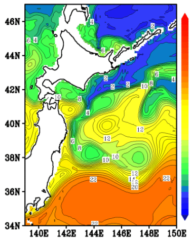
2022 年 11 月下旬/水温/平均値/100m (予報)
