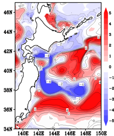
2022 年 11 月下旬/水温/平年差/100m (予報)
