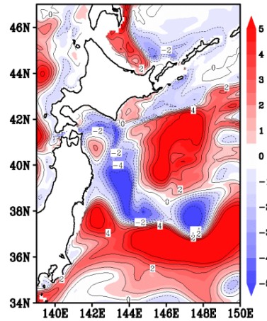
2022 年 11 月上旬/水温/平年差/100m (予報)
