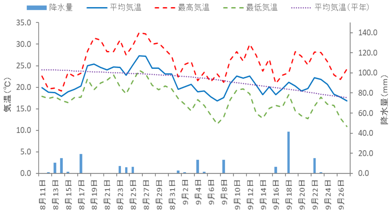
図1 8月11日から9月26日までの気温と降水量の推移 (アメダス地点：米山)
