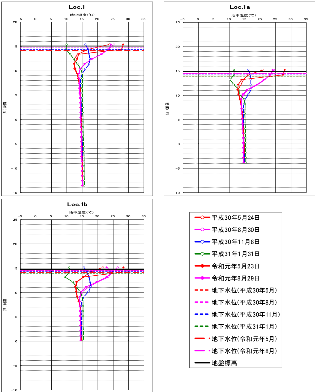
図 5-3 地中温度変化図 (地下水) ①
