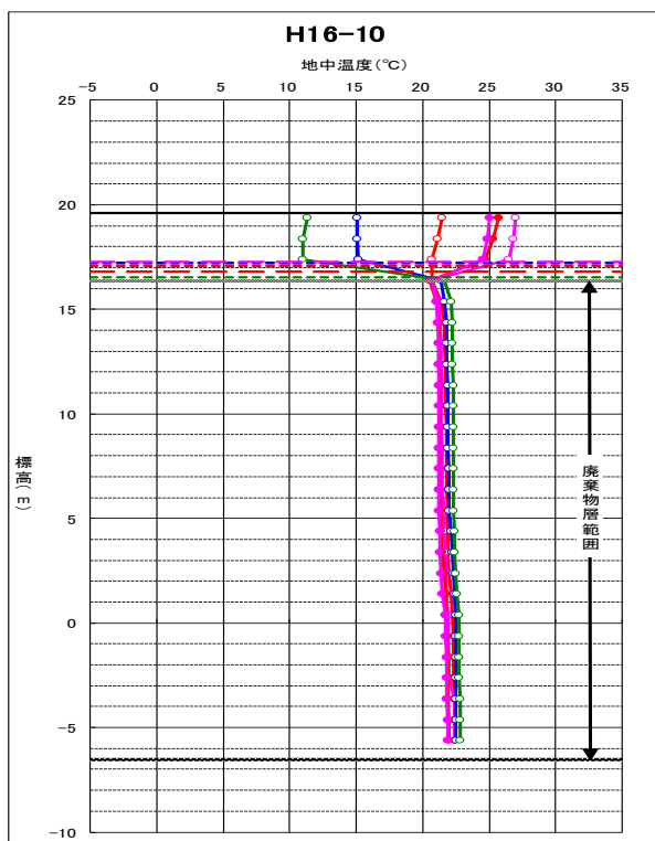
図 5-8 地中温度変化図 (浸透水) ②
