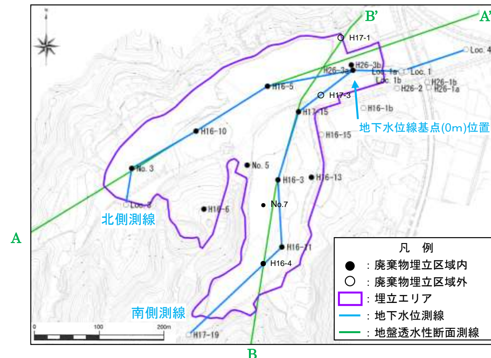
図5-14 令和元年度上半期のの上流側～下流側にかけての水位標高変化（平面図）
