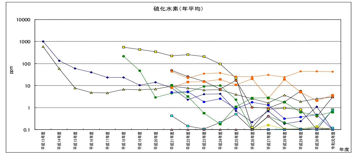
図 4-1 硫化水素（管頭下 1m で測定）※下图：対数表示
