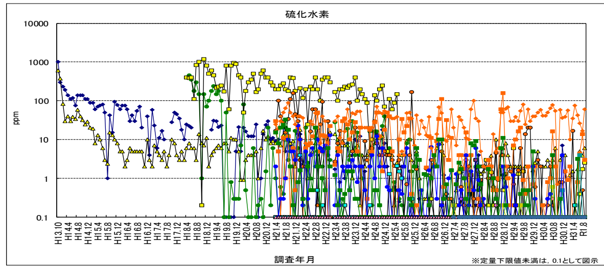
図 4-1 硫化水素（管頭下 1m で測定）※下图：対数表示
