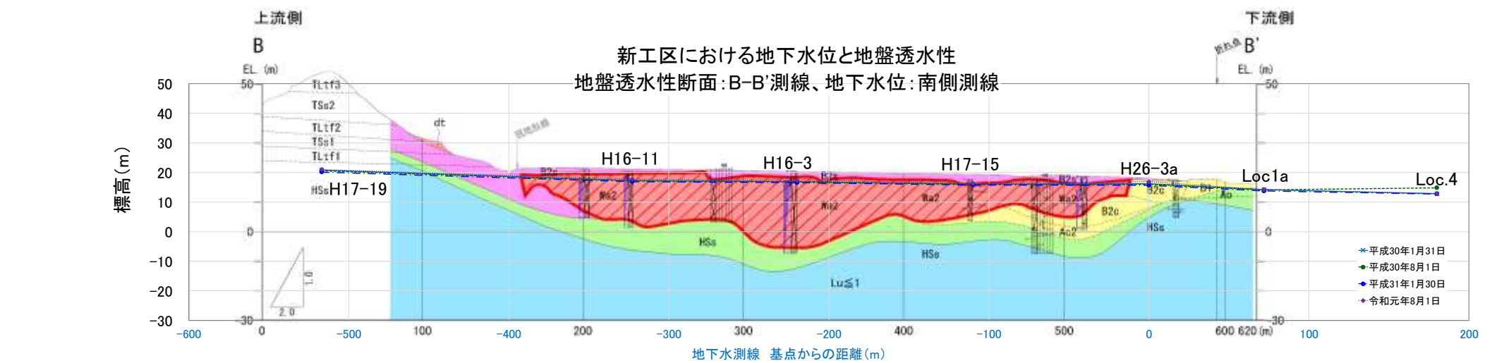
図5-13 令和元年度上半期のの上流側～下流側にかけての水位標高変化（地盤透水性断面図）
