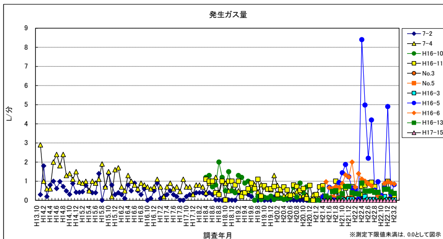
図 5-5 発生ガス量
