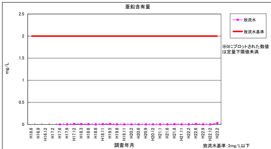
図 3-35 亜鉛含有量(放流水)
