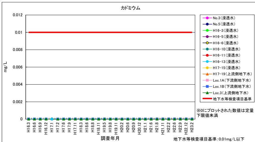
図 4-3 カドミウム（浸透水・地下水）
