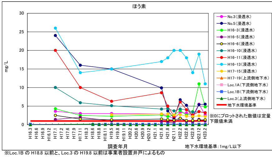
図 4-28 ほう素（浸透水・地下水）
