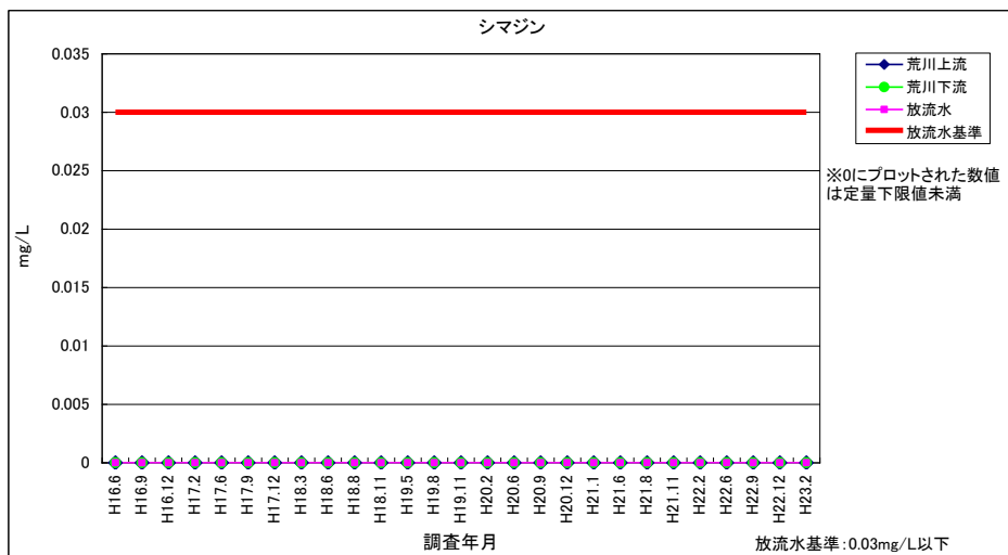
図 3-21 シマジン（放流水・河川水）
