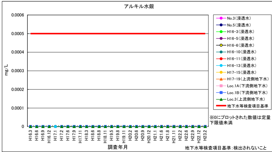
図 4-1 アルキル水銀（浸透水・地下水）
