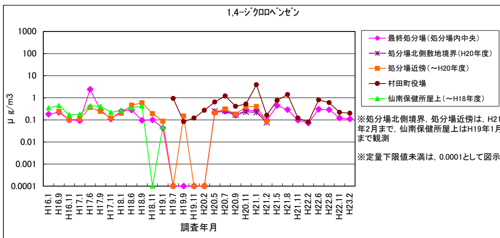
図 1-45 1,4-ジクロロベンゼン
