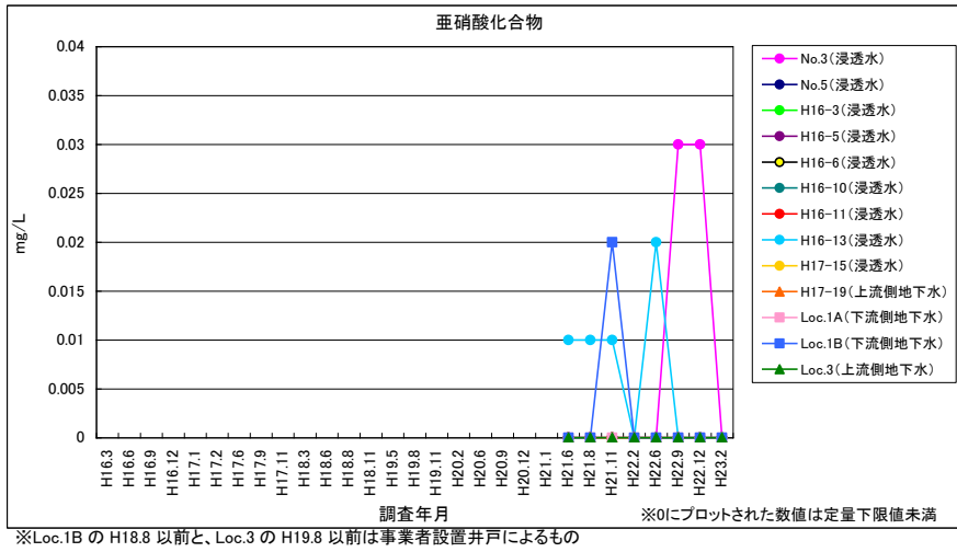
図 4-31 垂硝酸化合物（浸透水・地下水）
