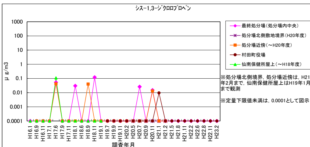
図 1-33 シス-1,3-ジクロロプロペン
