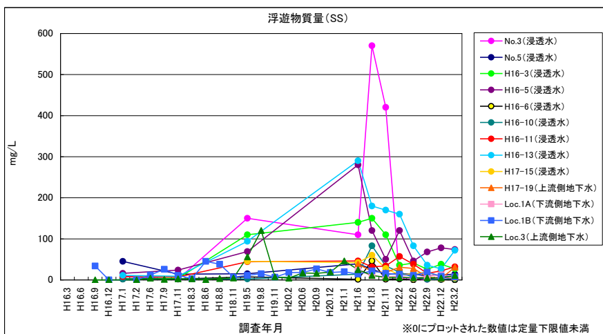
図 4-27 浮遊物質質量 (SS) (浸透水・地下水)
