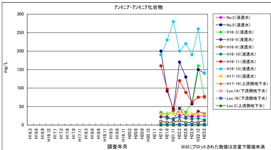
図 4-30 アンモニア、アンモニア化合物（浸透水・地下水）
