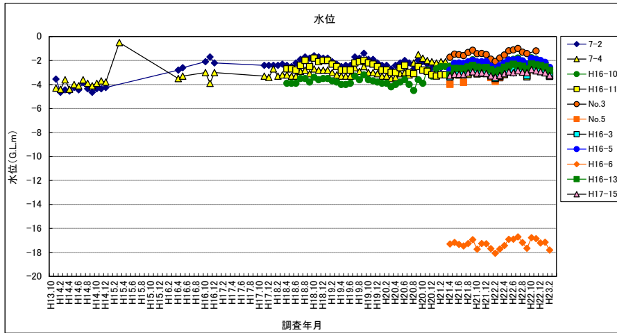
図 5-7 水位
