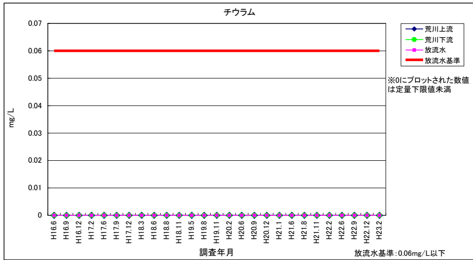
図 3-20 チウラム（放流水・河川水）
