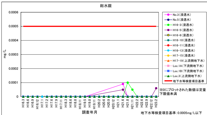
図 4-2 総水銀（浸透水・地下水）
