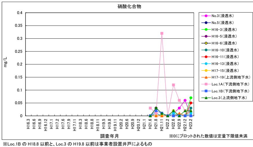
図 4-32 硝酸化合物（浸透水・地下水）
