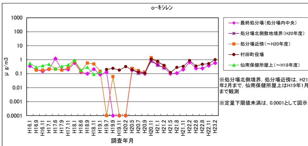
図 1-39 o-キシレン
