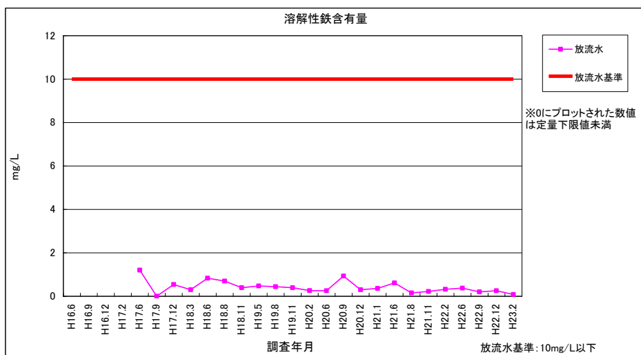
図 3-36 溶解性鉄含有量 (放流水)
