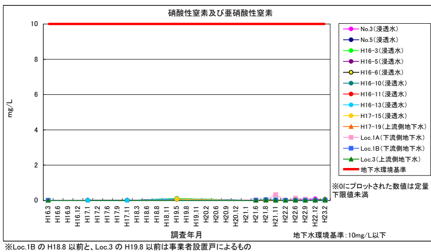
図 4-33 硝酸性窒素及び亜硝酸性窒素（浸透水・地下水）
