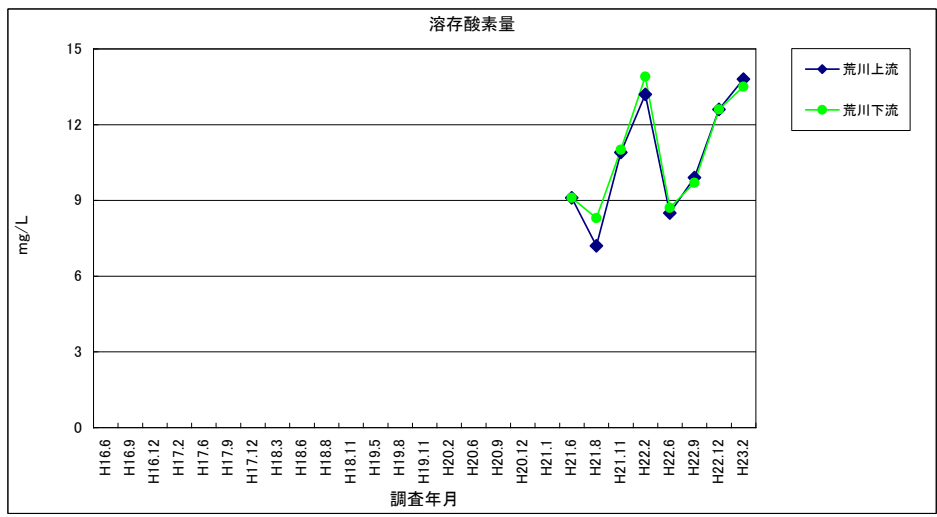
図 3-40 溶存酸素量 (河川水)
