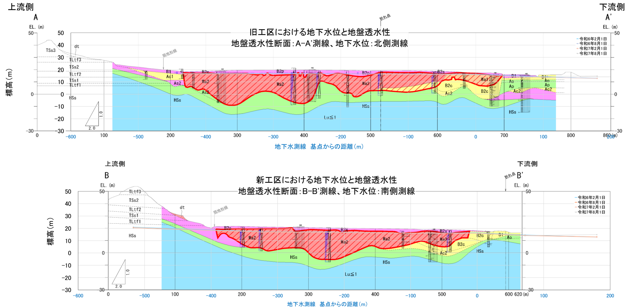
図 2-55 令和7年度上半期のの上流側～下流側にかけての水位標高変化（地盤透水性断面図）
