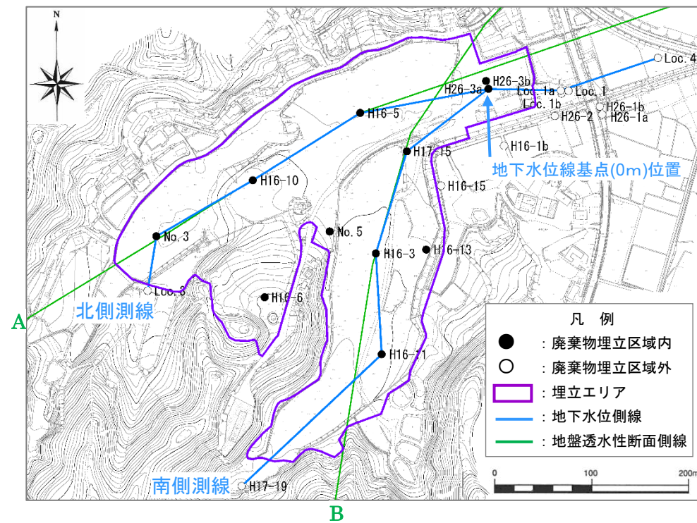
図 6-11 令和7年度上半期の北側側～南側側にかけての水位標高変化 (平面図)
