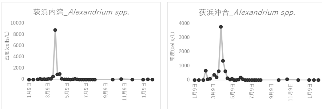
図 萩浜内湾・萩浜沖の麻痺性貝毒プランクトン密度の推移
