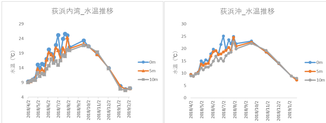
図 萩浜内湾・萩浜沖の水温の鉛直分布
