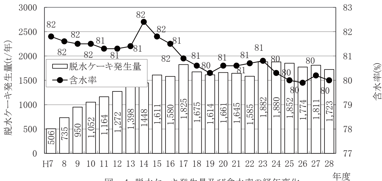
図-4 脱水ケーキ発生量及び含水率の経年変化 年度
