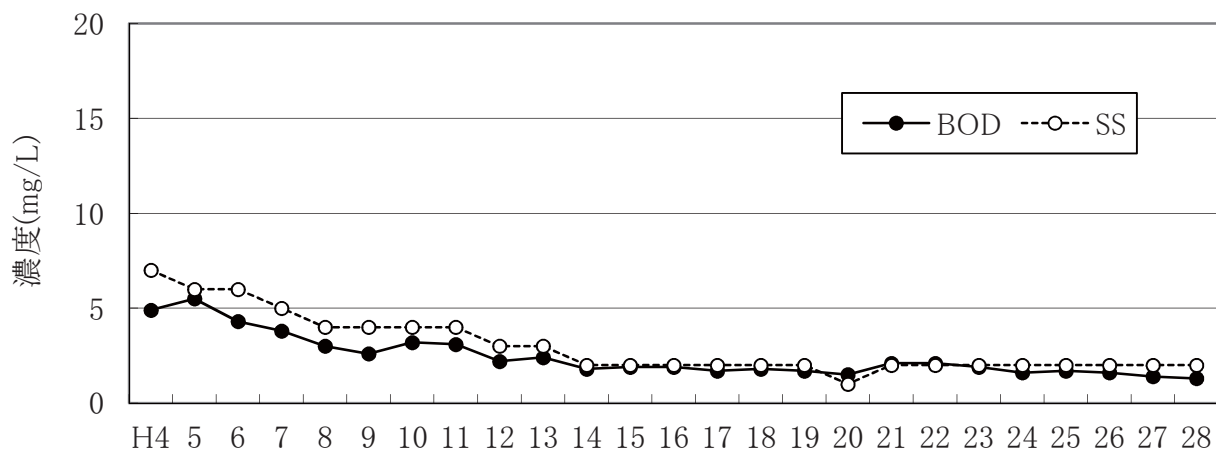
図-3 放流水の水質経年変化 年度
