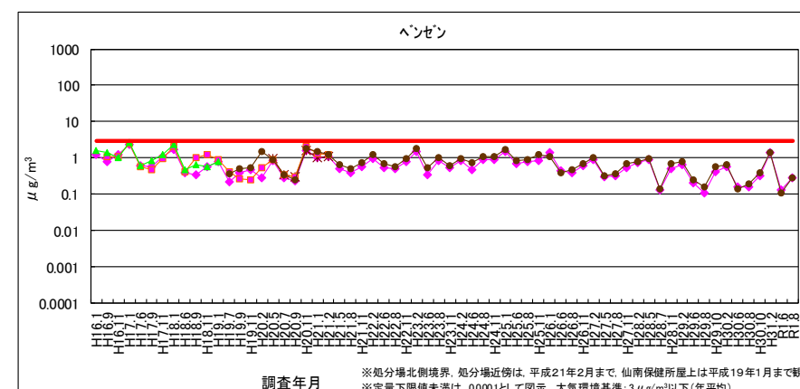
図 2-3 ベンゼン
