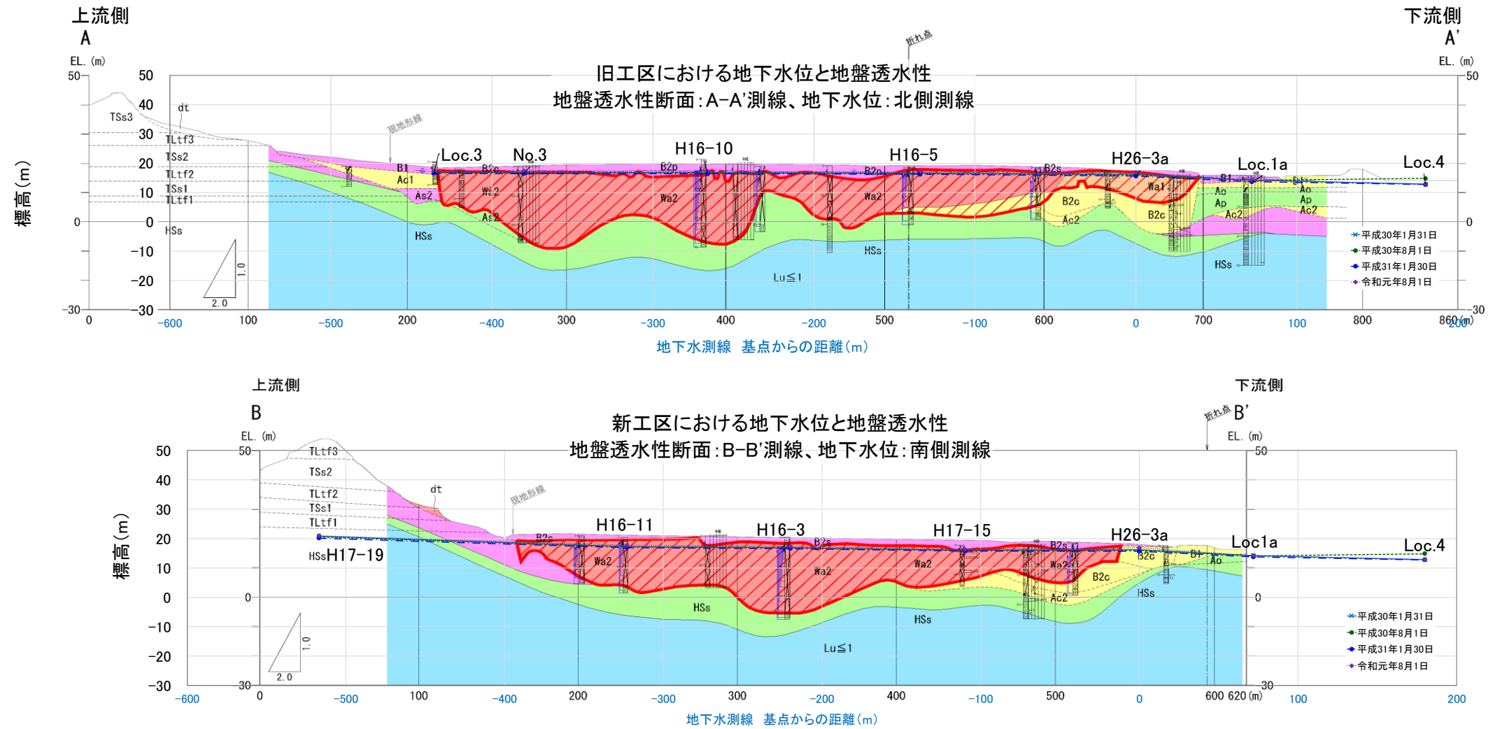
図2-59 令和元年度上半期の上流側～下流側にかけての水位標高変化（地盤透水性断面図）
