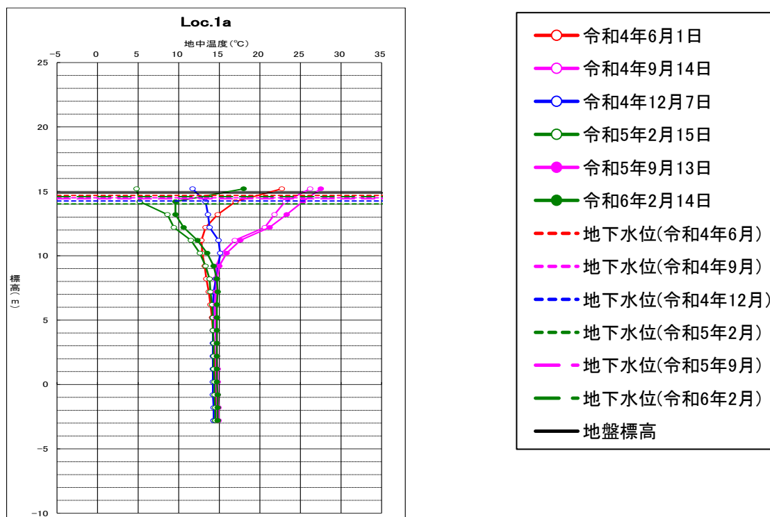
図 6-3 地中温度変化図（地下水）
