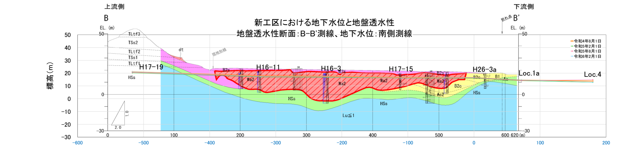
図 6-10 令和5年度下半期の上流側～下流側にかけての水位標高変化（地盤透水性断面図）
