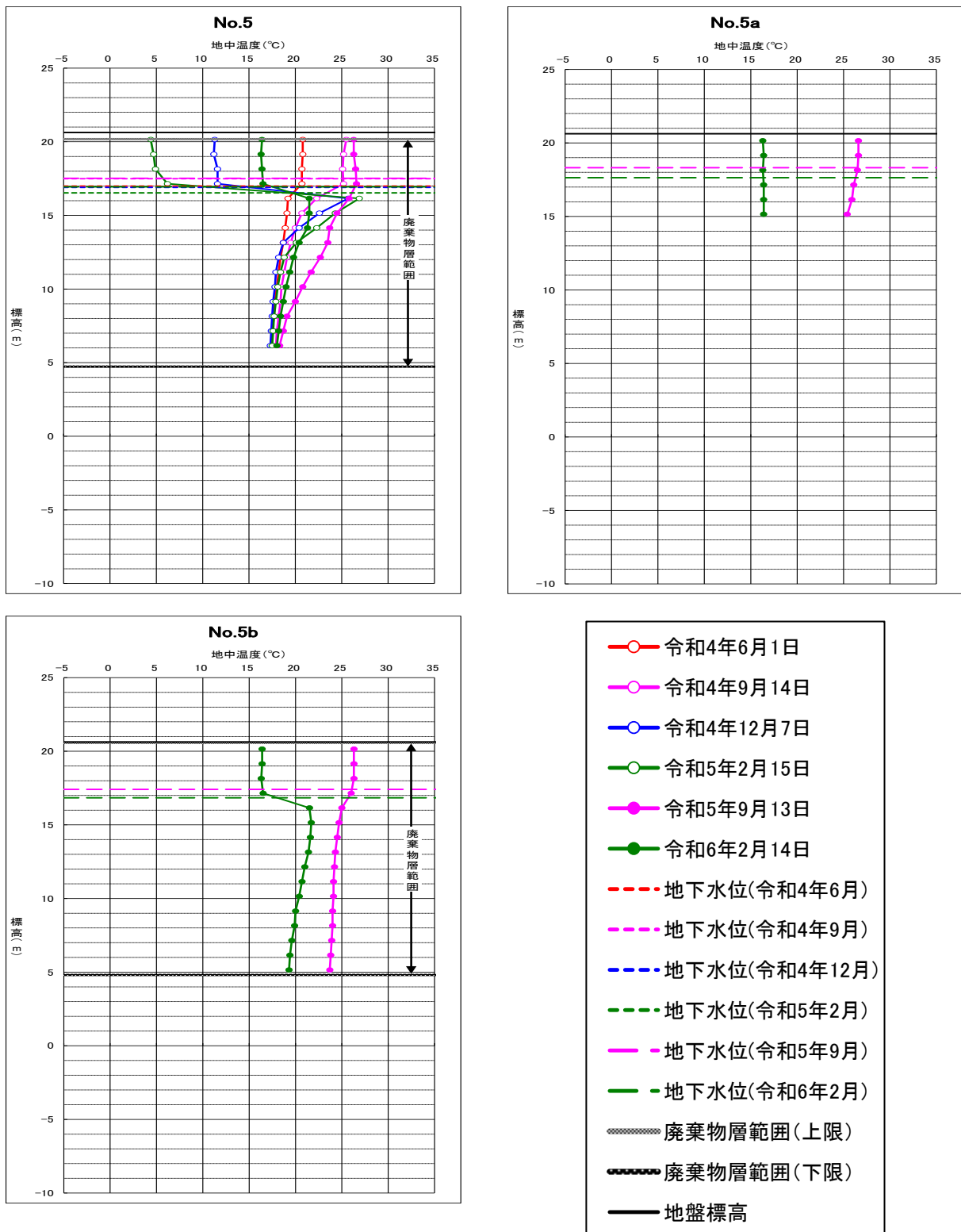
図 6-4 地中温度変化図(浸透水) ①
