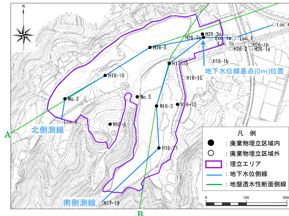
図 6-11 令和5年度下半期の上流側～下流側にかけての水位標高変化（平面図）
