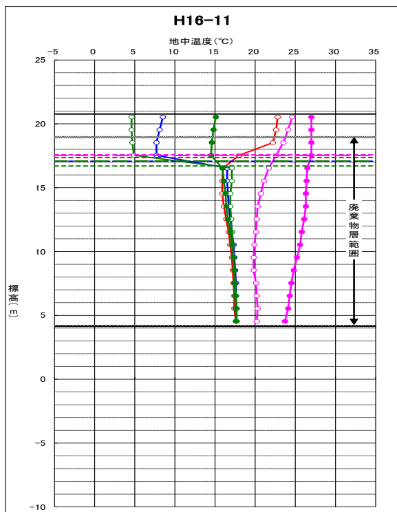
图 6-6 地中温度变化图 (浸透水) ③
