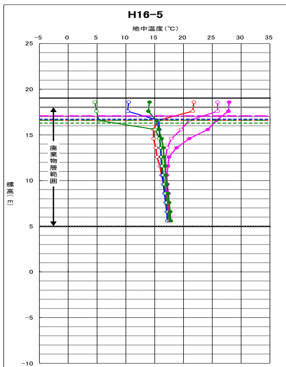
図 6-5 地中温度変化図（浸透水）②
