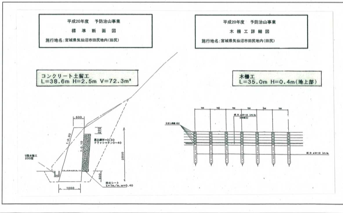
標準断面図，構造図 (1/100)
