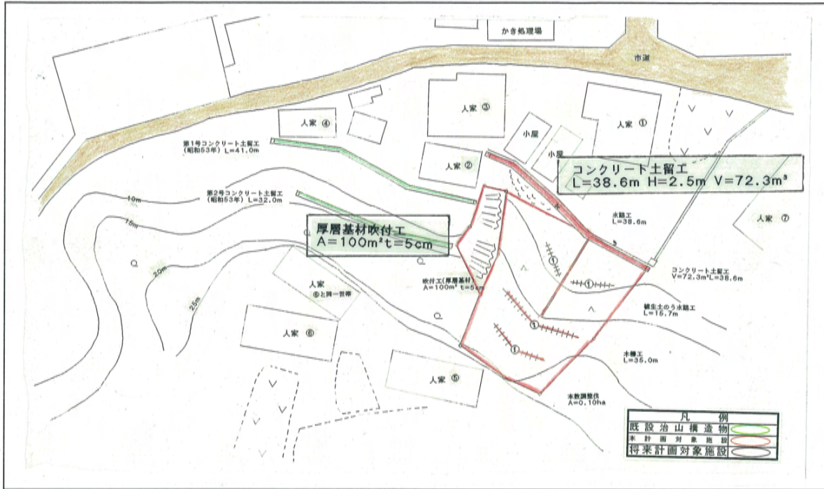
平面図 (1/1,000)
