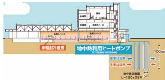
(庁舎の地中熱ヒートポンプシステムのしくみ) 役場の駐車場の下に、深さ100mの地中熱交換器が29本掘られています。
