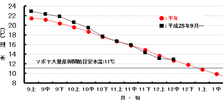
江ノ島旬平均水温
