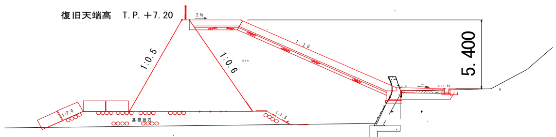
標準断面図 L1対応護岸
