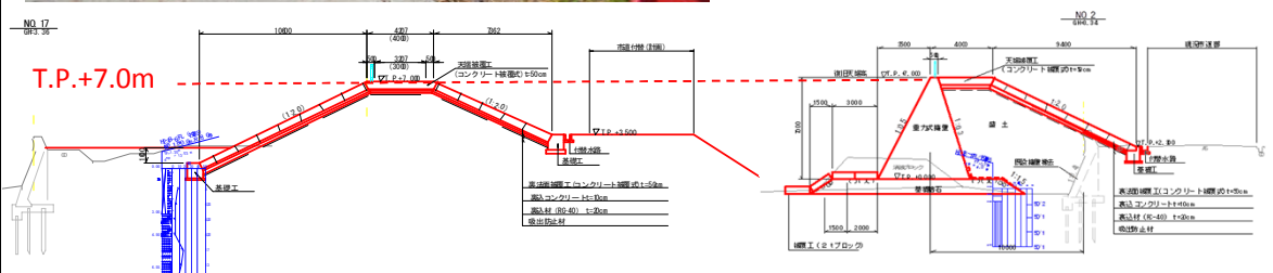
標準断面図 L1対応護岸工 (Standard Cross-section Diagram for L1 Seawall Work)
