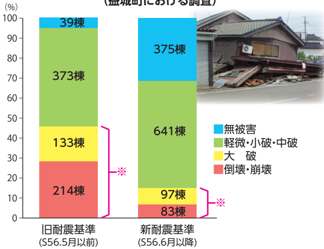
平成28年熊本地震の木造住宅被害 (益城町における調査)
