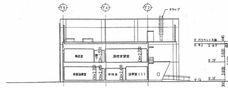
断面図
