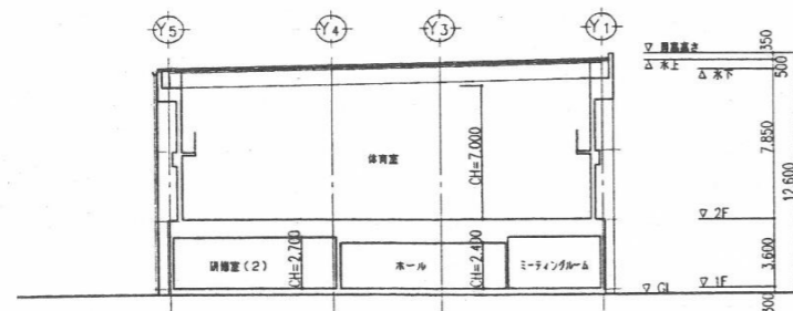
断面図
