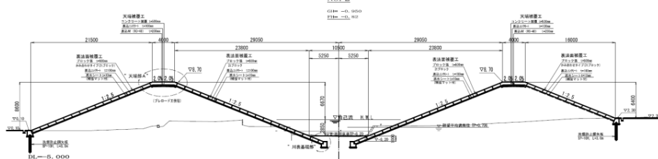
桜川復旧標準断面図
