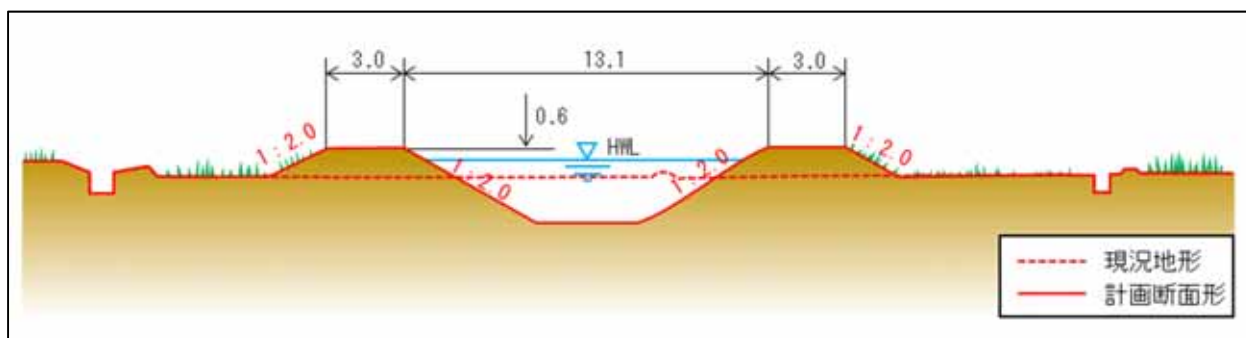
図 28 横断面図(多田川合流点から 4,200m)
