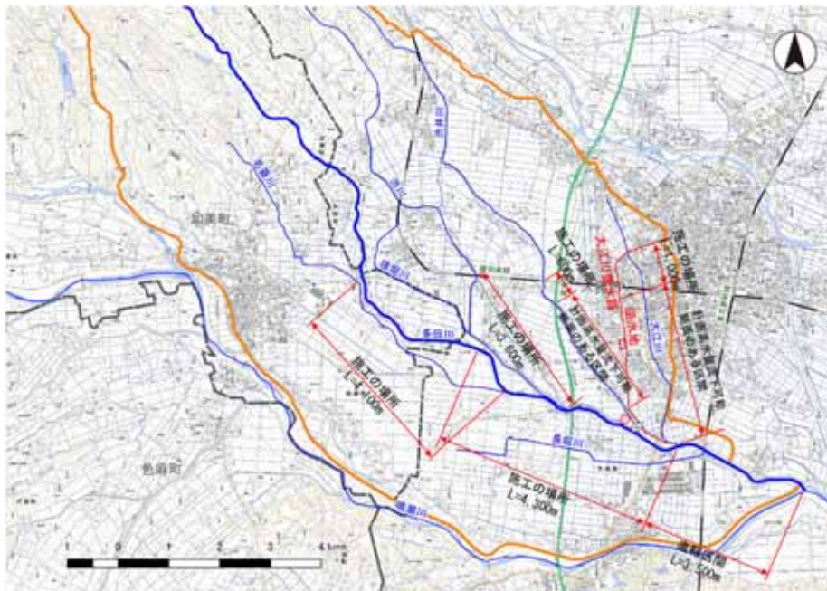
図 18 整備計画位置図
