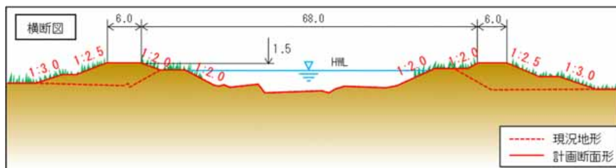
図 20 横断面図(多田川直轄管理境から 2,400m)
