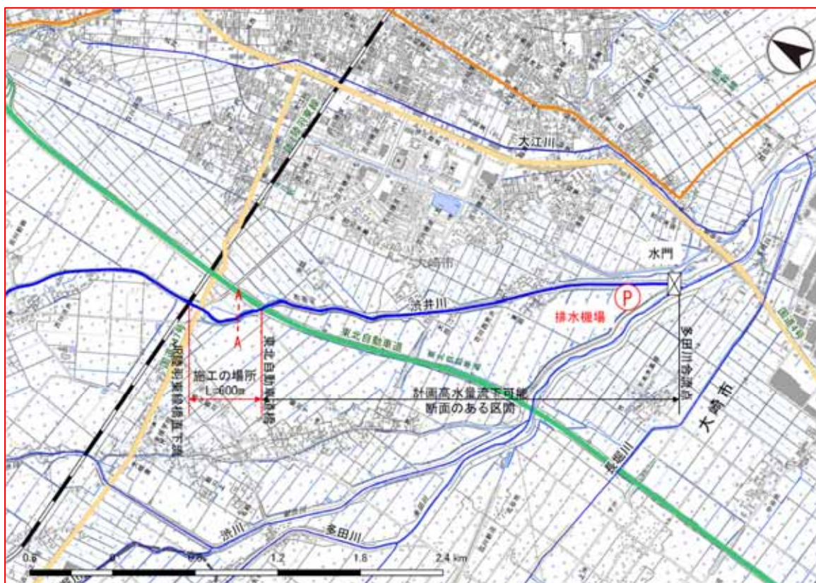
図 23 整備実施区間位置図
