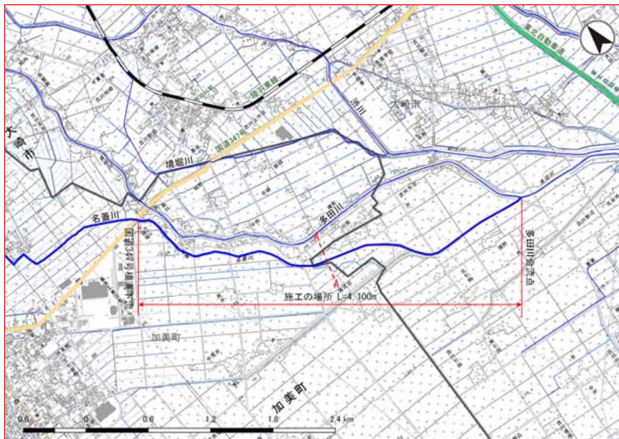
図 25 整備実施区間位置図
