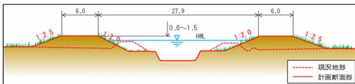
図 26 横断面図(多田川合流点から 2,000m)
