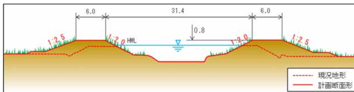
図 22 横断面図(多田川合流点から 2,200m)
