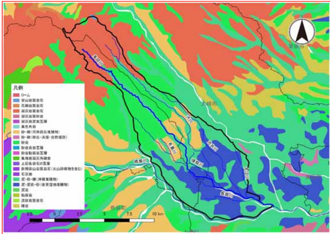
図 3 表層地層図
