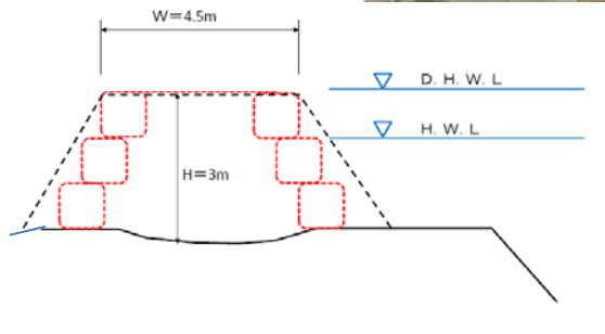
応急断面図
