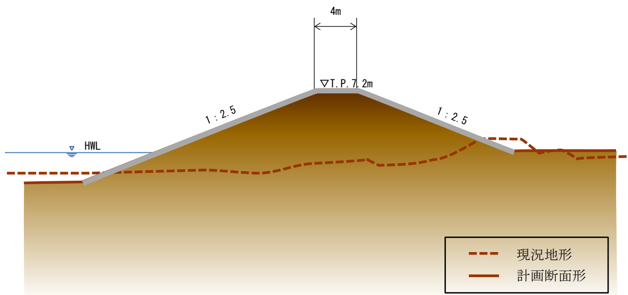
図 2-9 高潮、津波遡上に対応できる堤防整備イメージ 3
