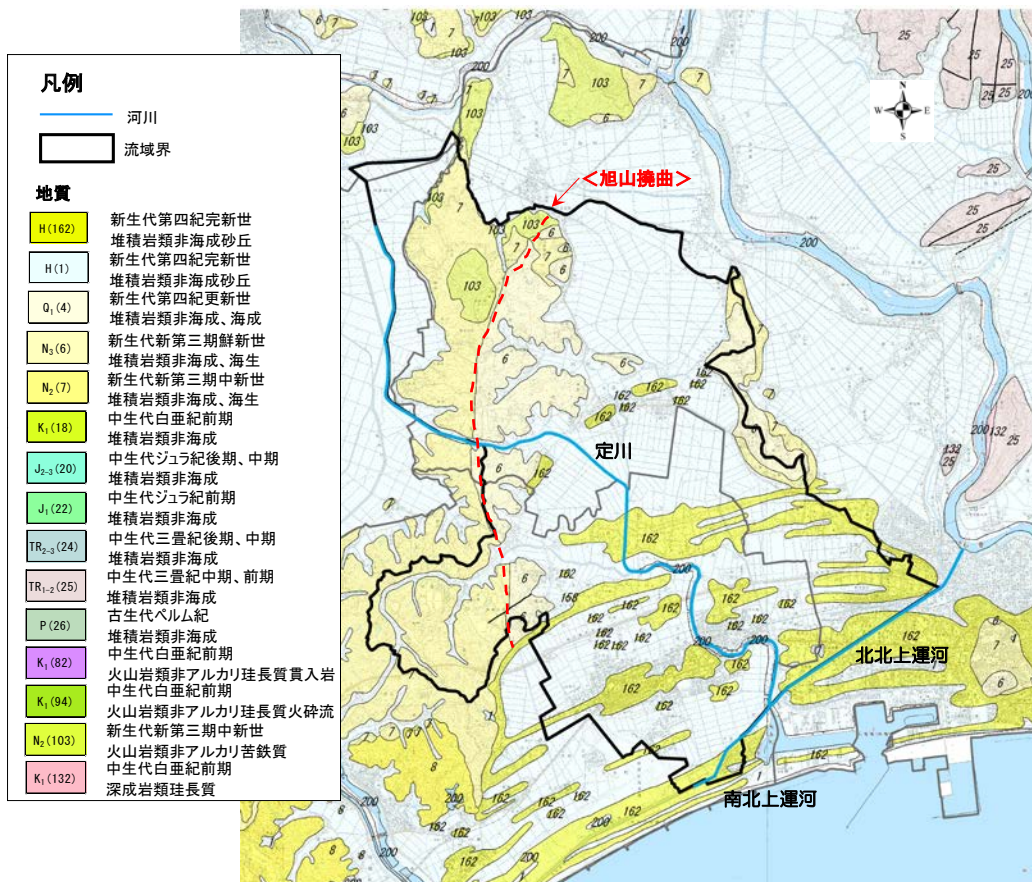
図 1-3 地質概略図
