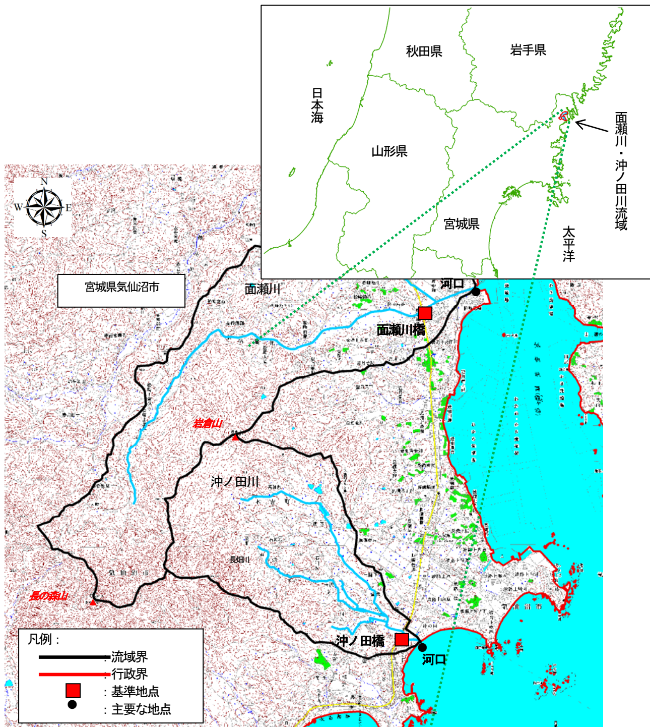
図 1-1 流域図
