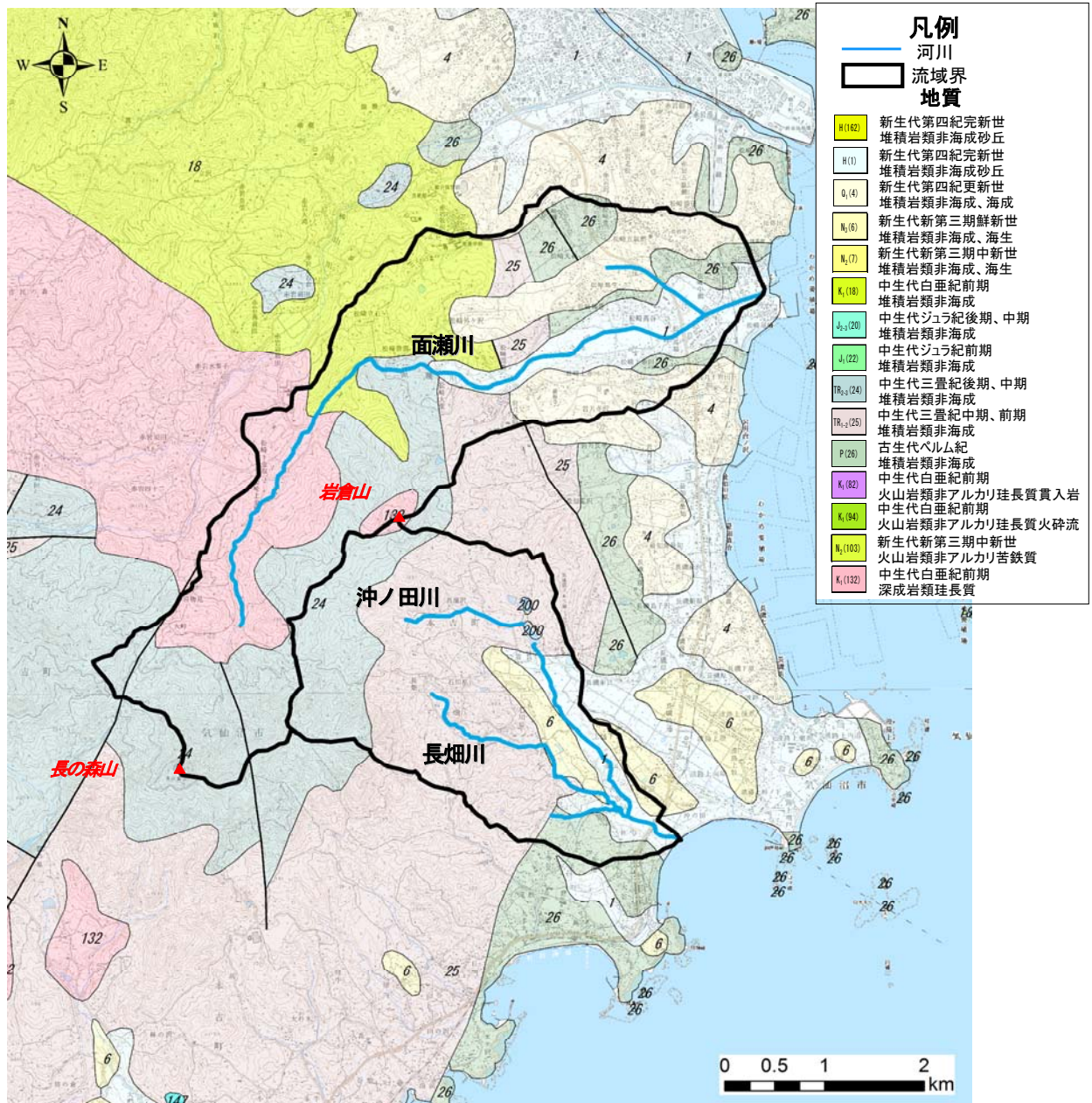
図 1-3 地質概略図
