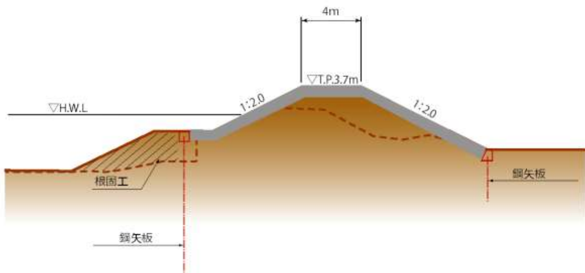
図 2-10 高潮、津波遡上に対応できる堤防整備イメージ 6
