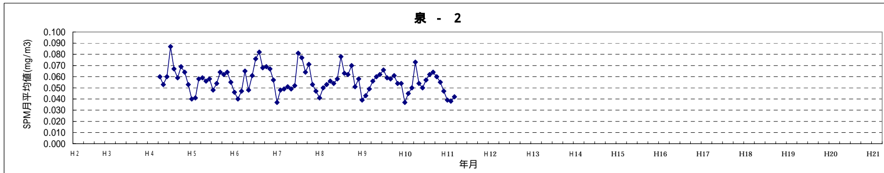
図3-1-3-(3) 浮遊粒子状物質濃度月平均値の経月変化 - ( 3 ) ( 自排局、H2~H20 )
