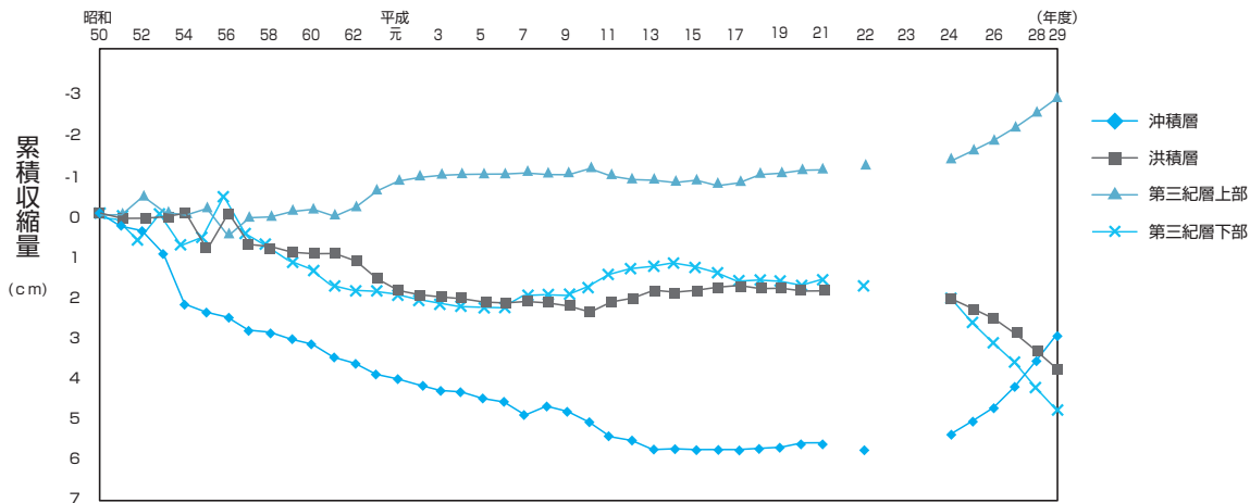
▲図3-4-1-27 苦竹地盤沈下観測井における地層収縮量の経年変化
